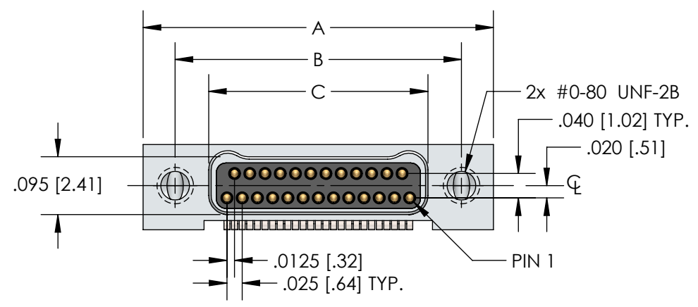
PLUG (PINS)
