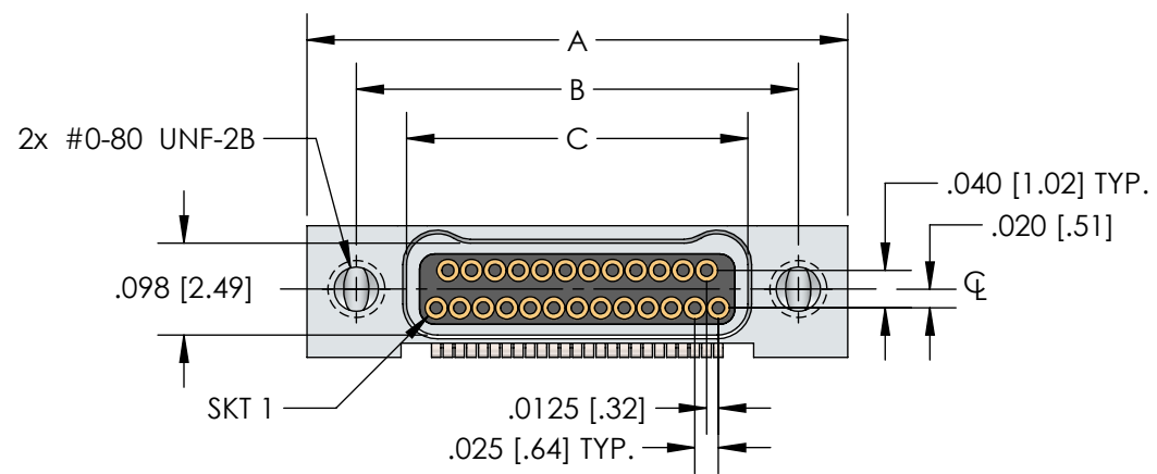
RECEPTACLE (SOCKETS)
